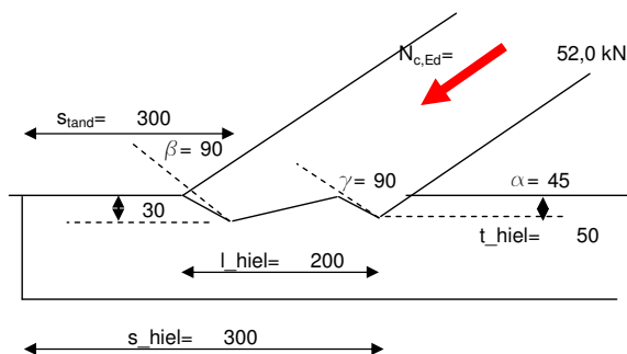
zie figuur NB4 - Voorbeeld van een hielverbinding
